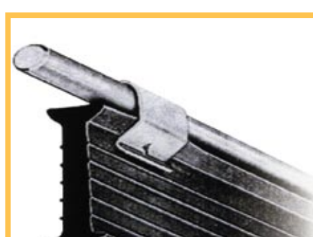
фиксация гидрошпонок при помощи механического крепежа
