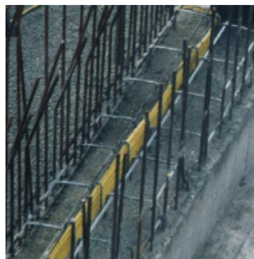
вспомогательные элементы из арматуры для крепления гидрошпонок
