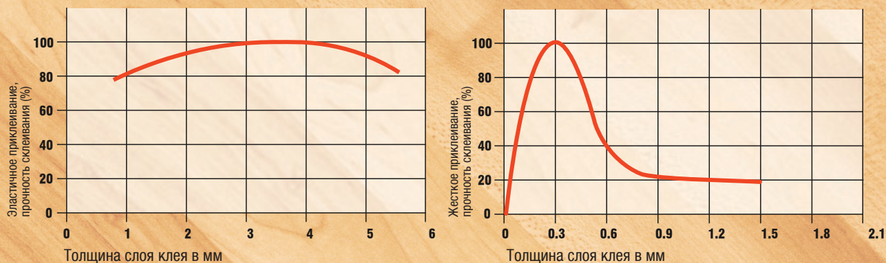
Рис.4: Влияние толщины слоя клея на прочность склеивания
