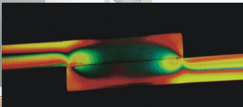
Рис.2а: Фотоупругая модель для анализа жестких клеев
