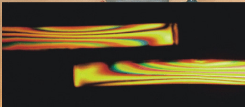
Рис.2б: Фотоупругая модель для анализа эластичных клеев
