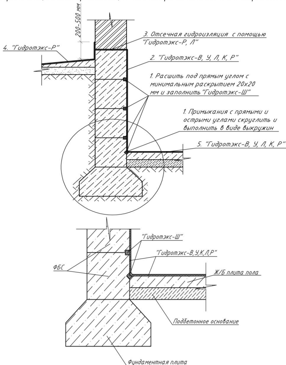
Рисунок 2: Устройство внутренней гидроизоляции подвала, выполненного из фундаментных блоков, с применением сухих дисперсных строительных гидроизоляционных проникающих капиллярных смесей ТМ «Гидротэкс»
