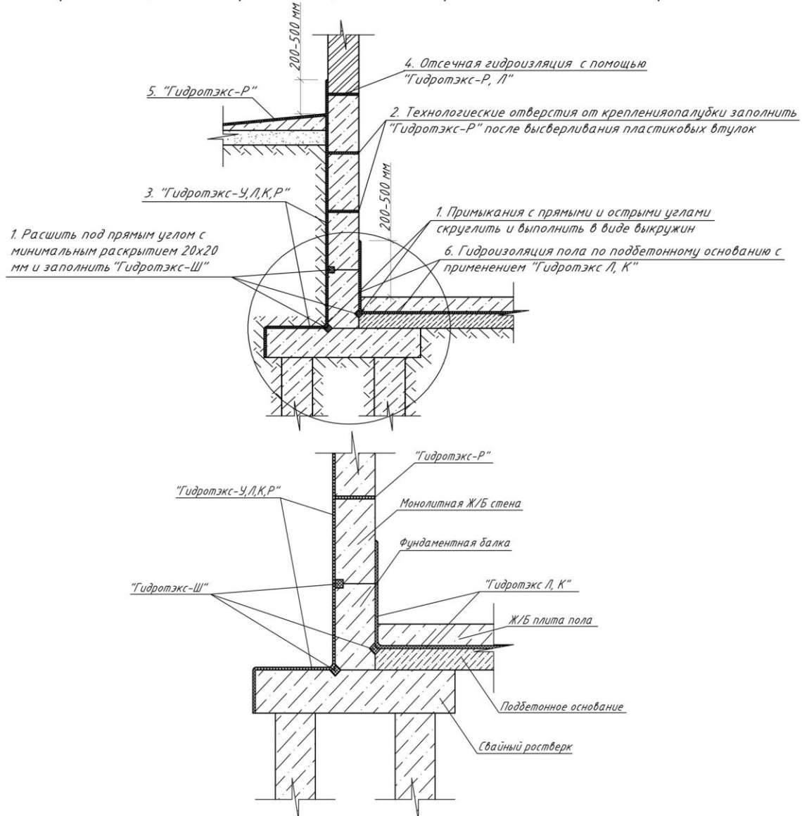
Рисунок 3: Устройство внешней гидроизоляции подвала, выполненного из монолитного Ж/Б, с применением сухих дисперсных строительных гидроизоляционных проникающих капиллярных смесей ТМ «Гидротэкс»
