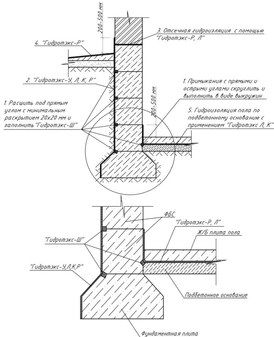
Рисунок 1: Устройство внешней гидроизоляции подвала выполненного из фундаментных блоков, с применением сухих дисперсных строительных гидроизоляционных проникающих капиллярных смесей ТМ «Гидротэкс»
