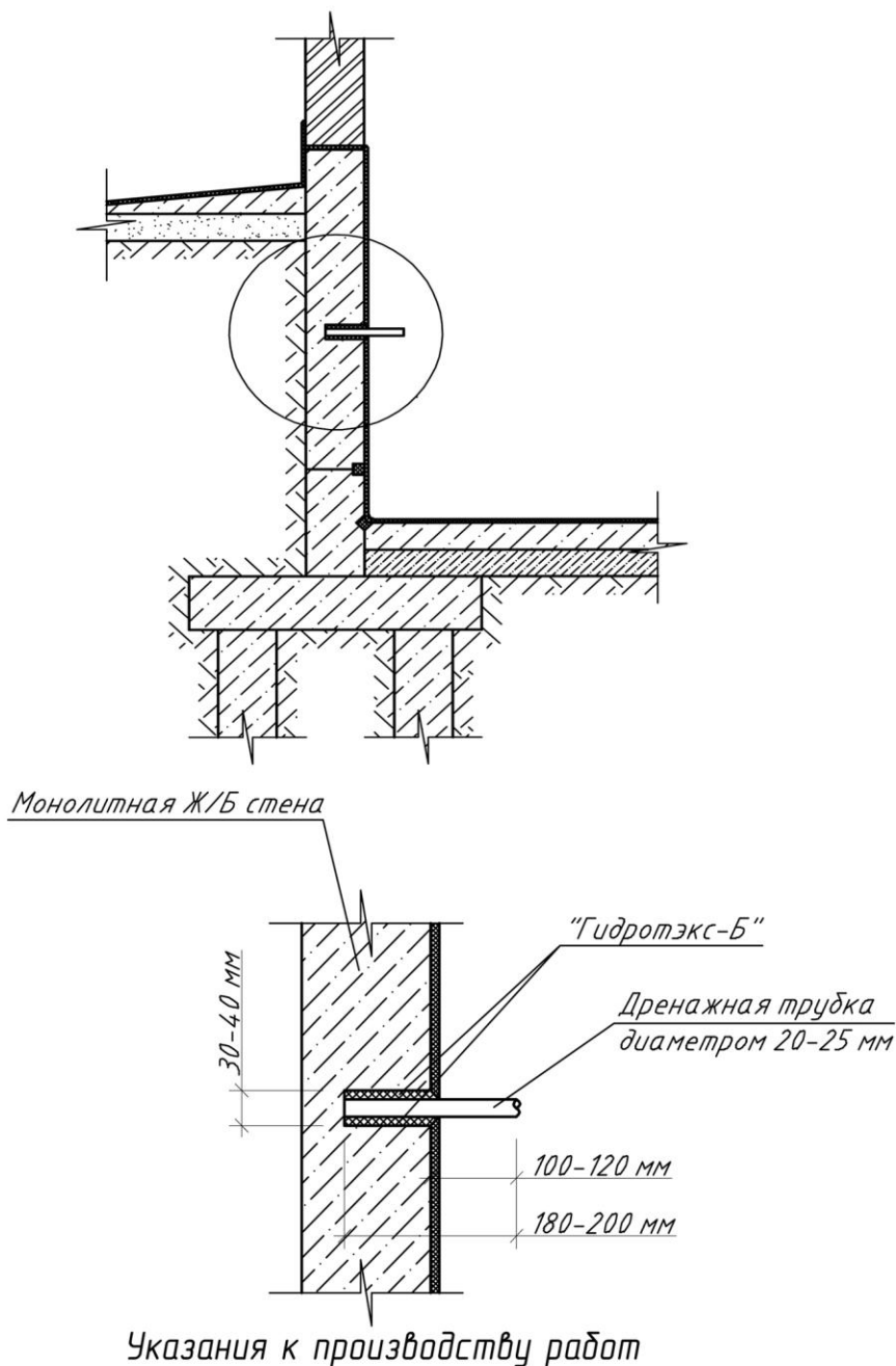
Рисунок 6: Разделка мест напорных течей и устройство дренажа, с применением сухих дисперсных строительных гидроизоляционных проникающих капиллярных смесей ТМ «Гидротэкс»
