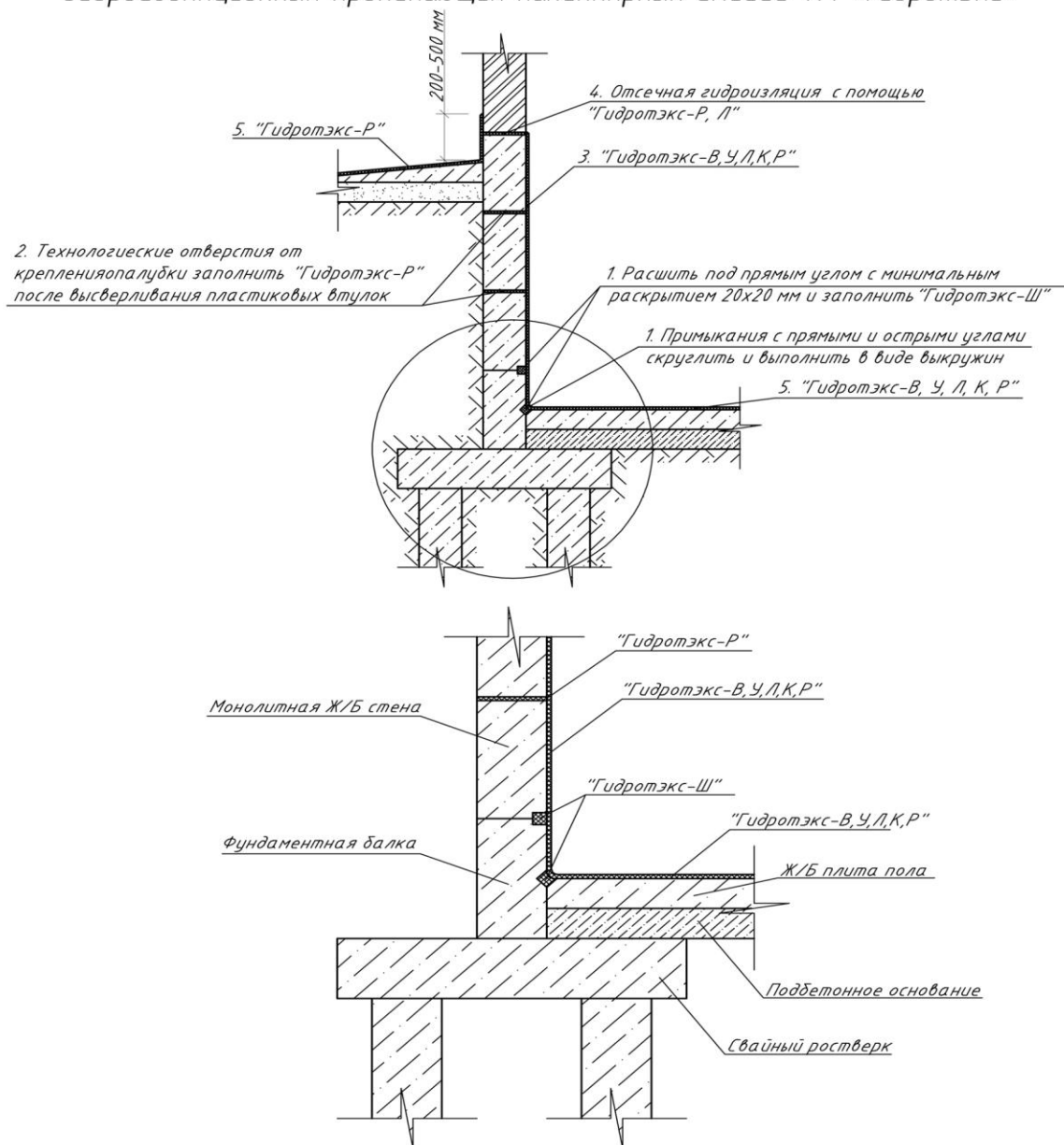
Рисунок 4: Устройство внутренней гидроизоляции подвала, выполненного из монолитного Ж/Б, с применением сухих дисперсных строительных гидроизоляционных проникающих капиллярных смесей ТМ «Гидротэкс»
