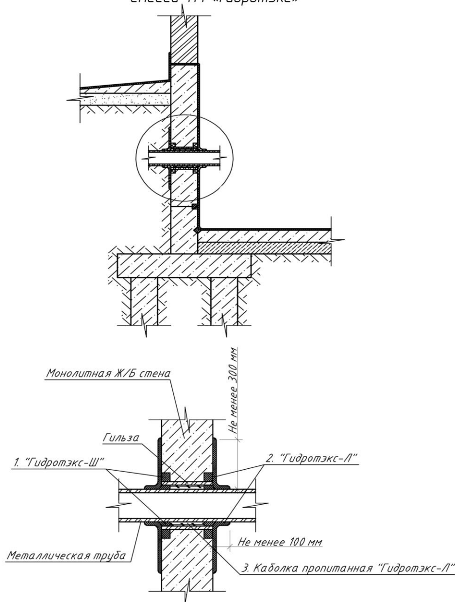
Рисунок 5: Устройство гидроизоляции вводов коммуникаций, с применением сухих дисперсных строительных гидроизоляционных проникающих капиллярных смесей ТМ «Гидротэкс»
