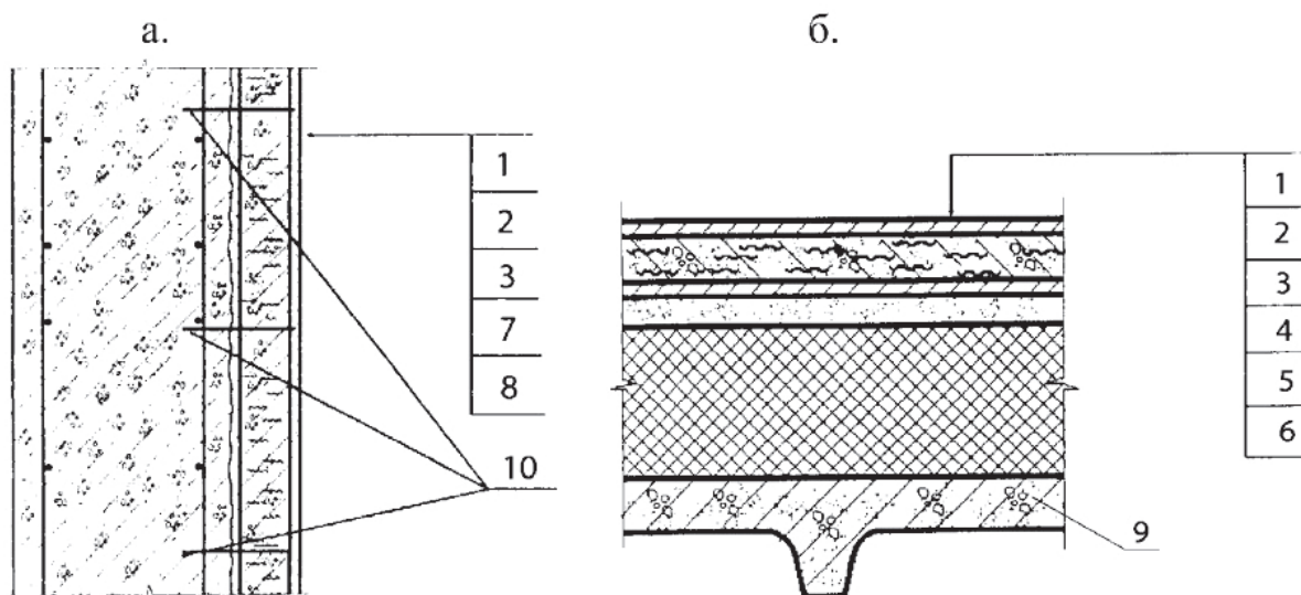
Рис. 6.3 – Торкретирование откосов и дна каналов
