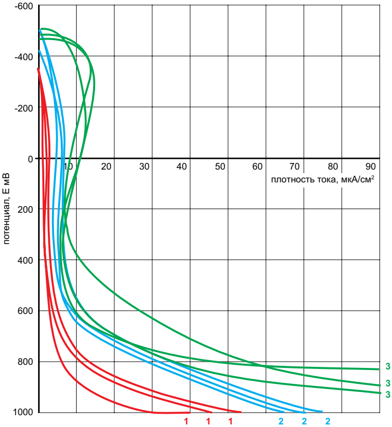
Рис. 2.2. Анодные поляризационные кривые стали с покрытием Mapefer 1K после 3-х месяцев испытаний в режиме: 1 — переменное увлажнение водой и высушивание; 2 — переменное увлажнение 5%-ным раствором NaCl и высушивание; 3 — переменное увлажнение водой и высушивание в бетоне с хлоридами (CaCl 2 ).
