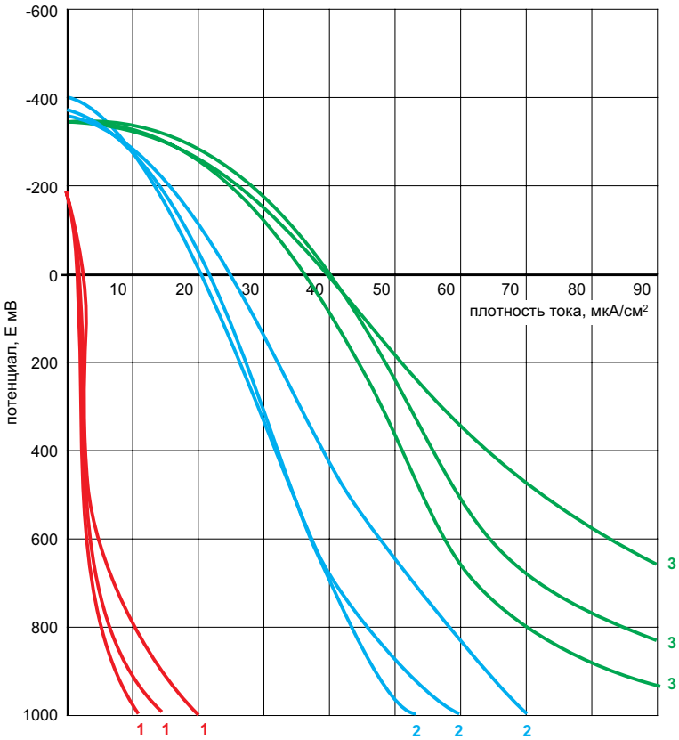
Рис. 2.2. Анодные поляризационные кривые стали без покрытия после 3-х месяцев испытаний в режиме: 1 — переменное увлажнение водой и высушивание; 2 — переменное увлажнение 5%-ным раствором NaCl и высушивание; 3 — переменное увлажнение водой и высушивание в бетоне с хлоридами (CaCl 2 ).
