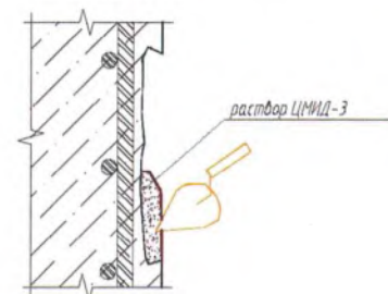
Поз. 6. Заполнение полости в три слоя композицией "ЦМИД-3" на глубину до 100 мм и площадью до 1 м 2
