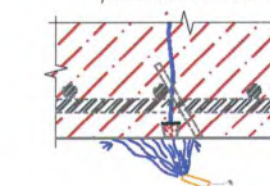
Поз 8. Инъектирование трещины раствором ЦМИД-СМ
