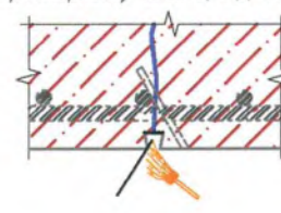
Рисунок В.2 – Герметизация трещин.
