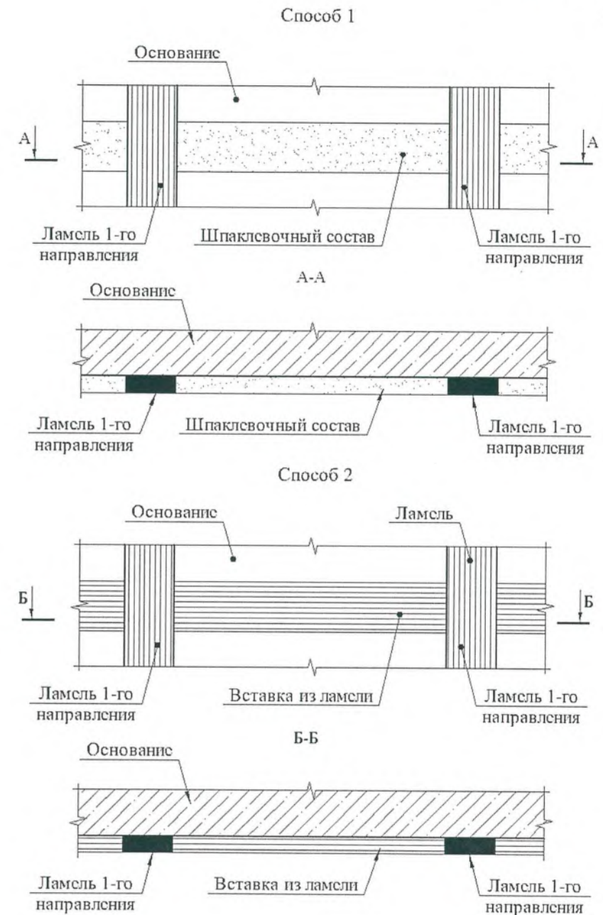
Рисунок Г.2 – Выравнивание основания под укладку ламелей во втором направлении
