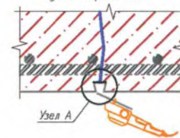
Поз 2. Сверление отверстий
