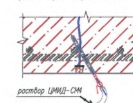
Поз 8. Инъектирование трещины раствором ЦМИД-СМ
