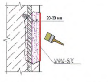
Рисунок В.1 – Ремонт участков с поверхностными дефектами бетона глубиной от 1 до 5 см и площадью до 1 м 2 без обнажения арматуры.
