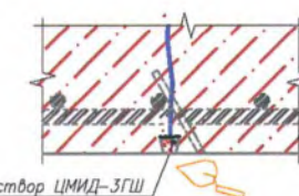
Поз 6. Зачеканка штрабы раствором ЦМИД-3ГШ
