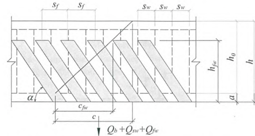
Рисунок 6 – Схема усилий при расчете железобетонных элементов с внешним армированием из полимерных композитов по наклонному сечению на действие поперечных сил
