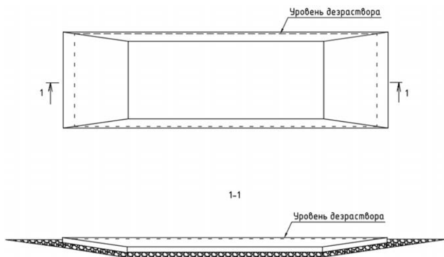
Рисунок 4.4.4.2 – Схема въездного дезбарьера без подогрева дезраствора
