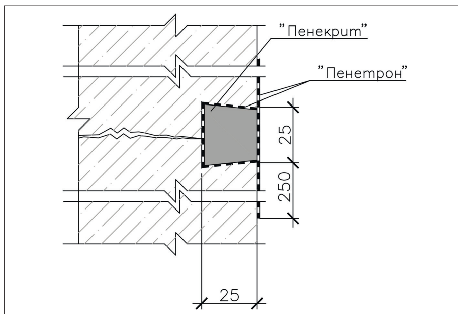
Рисунок 8.4. Схема ремонта и гидроизоляции сухих и влажных (без водонаполнения) статических трещины и швов бетонирования
