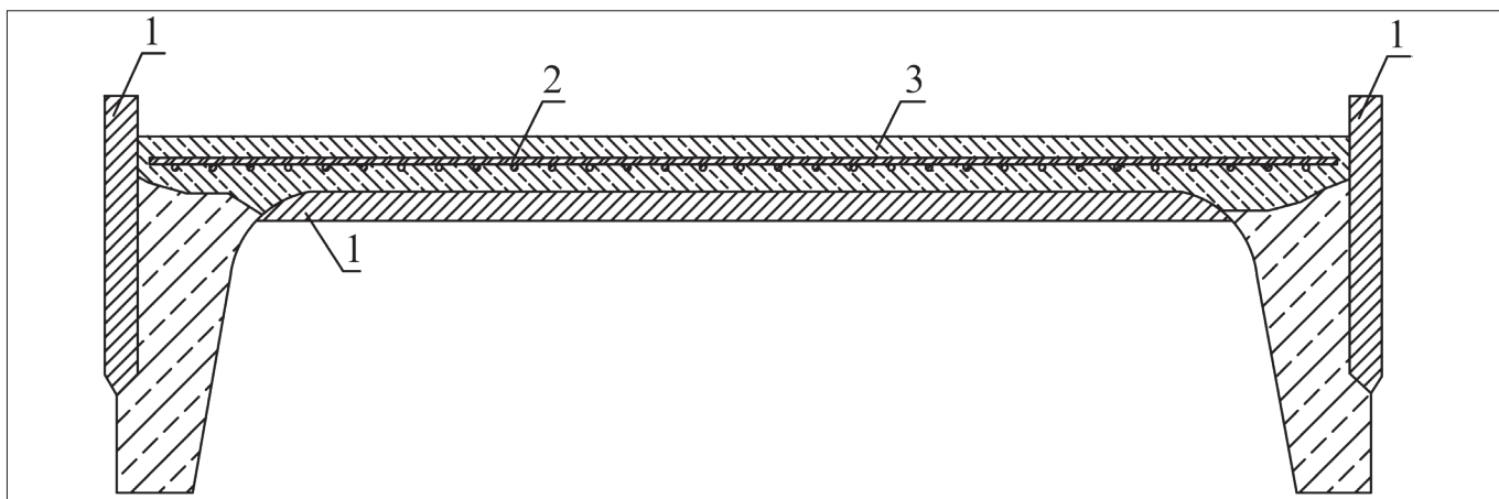
Рисунок 18 – Восстановление плиты в сжатой зоне
