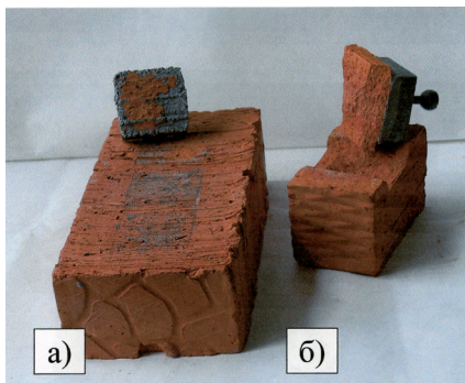
Рис. 3. Характер разрушения при испытании на адгезионную прочность а) 50% разрушения по контакту; б) разрушение по телу кирпича.
