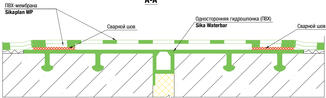
A-A
